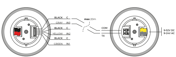
[Fig.2 / Abb.2] Schema di collegamento per ingresso 'smart sensor' (ver. MULTI/SPACE) Wiring diagram for 'smart sensor' (ver. MULTI/SPACE) Anschlusssschema für Eingang 'intelligenter Sensor' (ver. MULTI/SPACE) Esquema de conexión para la entrada 'smart sensor' (ver. MULTI/SPACE)
