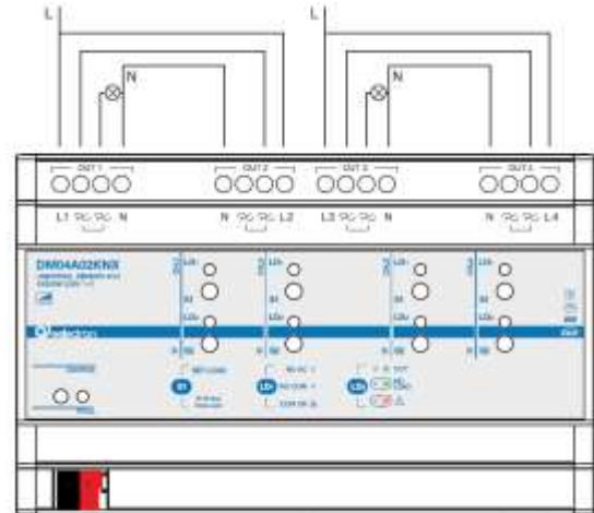
Schema di collegamento con canali abbinati
