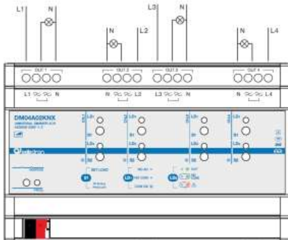
Schema di collegamento con canali indipendenti
