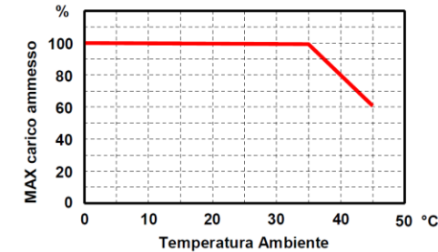
Fig. 1 - Declinamento del carico massimo ammesso in funzione della temperature ambiente:
