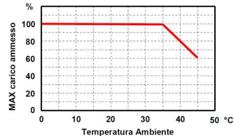
Fig. 1 - Declassamento del carico massimo ammesso in funzione della temperatura ambiente:
